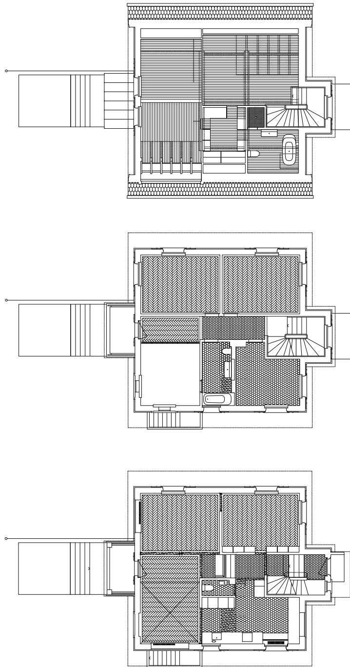
Grundrisse Dachgeschoss, 1. Obergeschoss, Erdgeschoss (v.o.n.u.)
